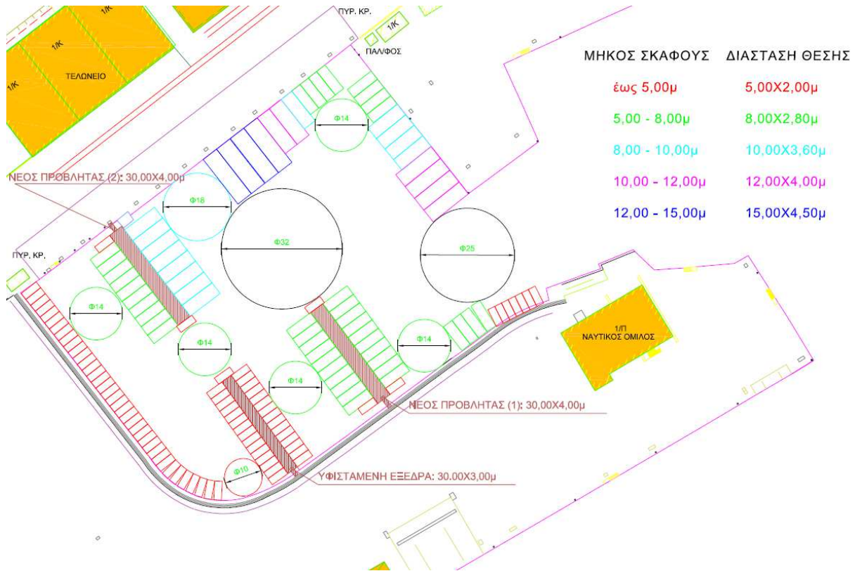
Σχήμα 3: Χωροδιάταξη προτεινόμενων πλωτών προβλητών - κυματοθραυστών μόνιμης χρήσης και ενδεικτική διάταξη θέσεων ελλιμενισμού
