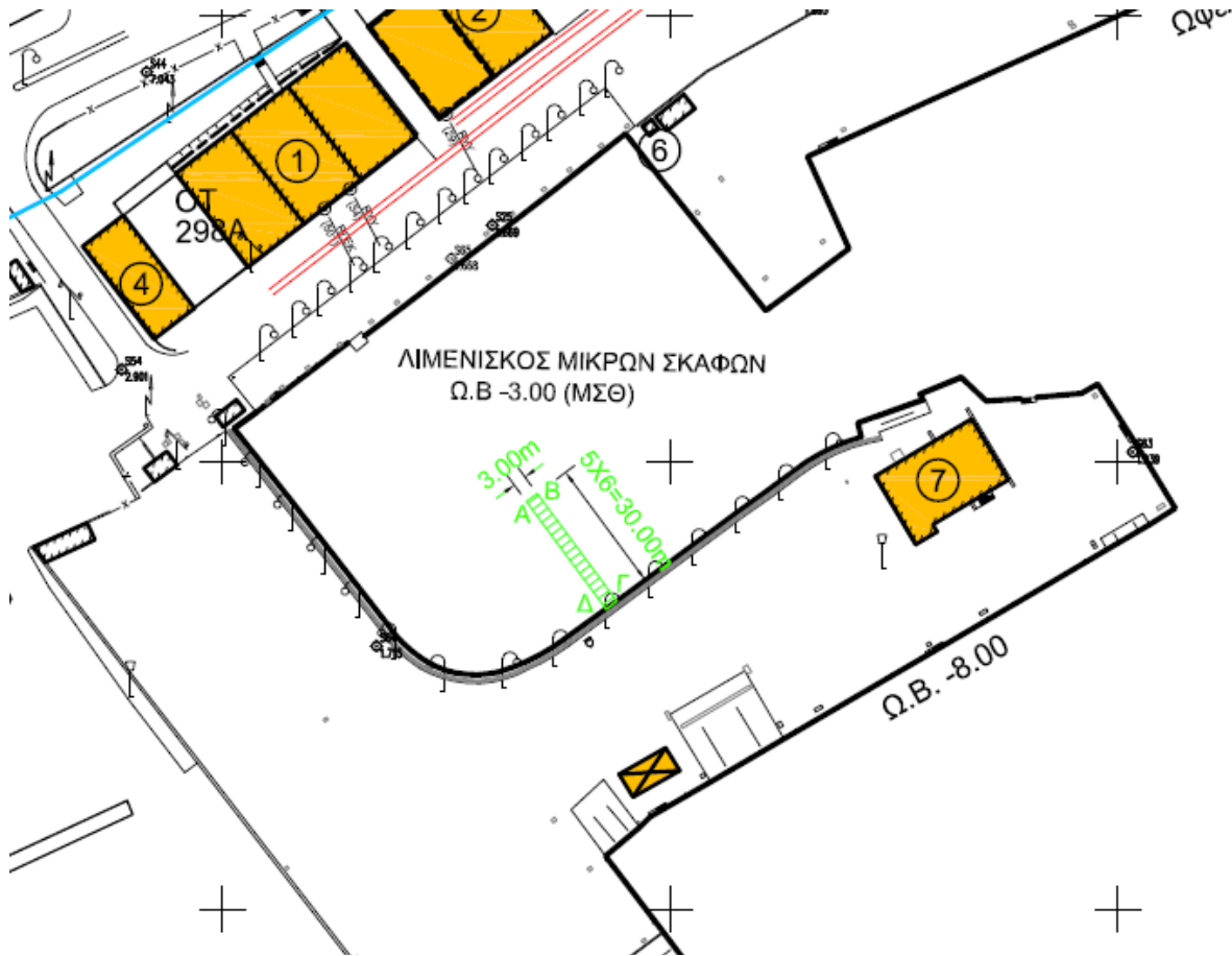
Σχήμα 2: Λιμενίσκος μικρών σκαφών λιμένα Αλεξανδρούπολης (με πράσινο χρώμα η υφιστάμενη θέση πλωτής εξέδρας εποχιακής χρήσης)
